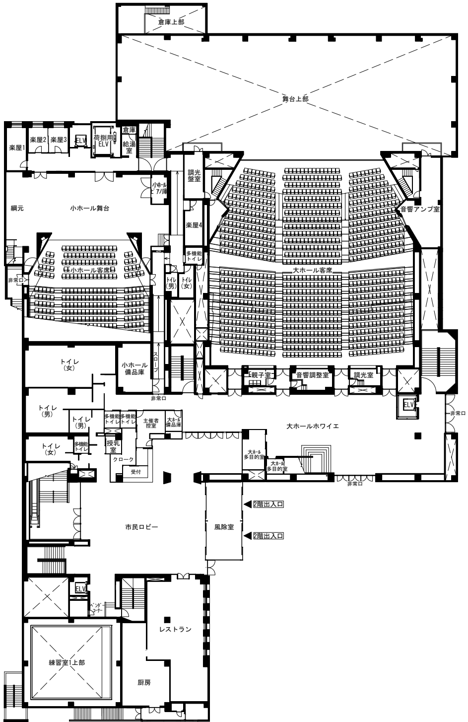
2階平面図
