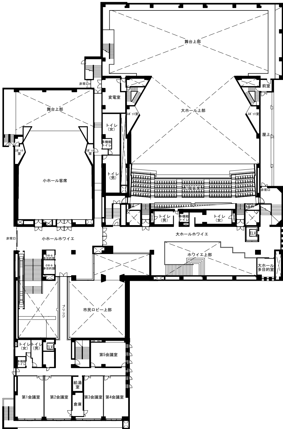
3階平面図
